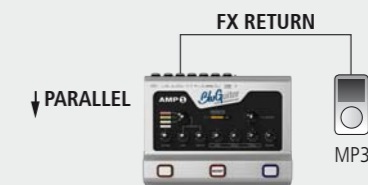
Abb. 4 MP3-Player im parallelen Mode
