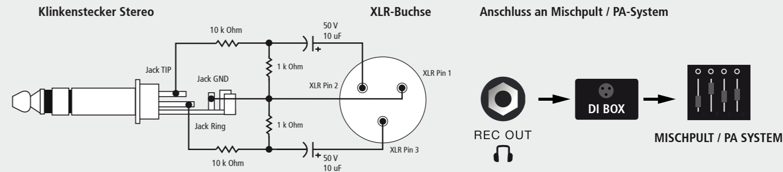
Abb. 1: Schaltplan für den Bau eines Adapters zum Anschluss an einen Mikrofoninput - mit Protection gegen Phantompower.
