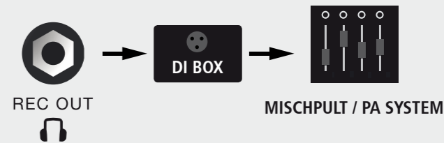
Abb. 2: Anschlussreihenfolge
