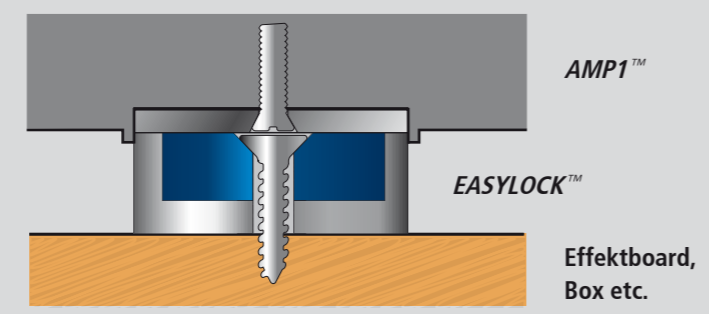
EASYLOCK™ Befestigung mit einer Holzschraube
