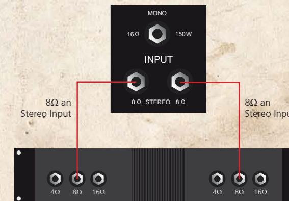
Stereo Endstufe / Gitarrenverstärker
